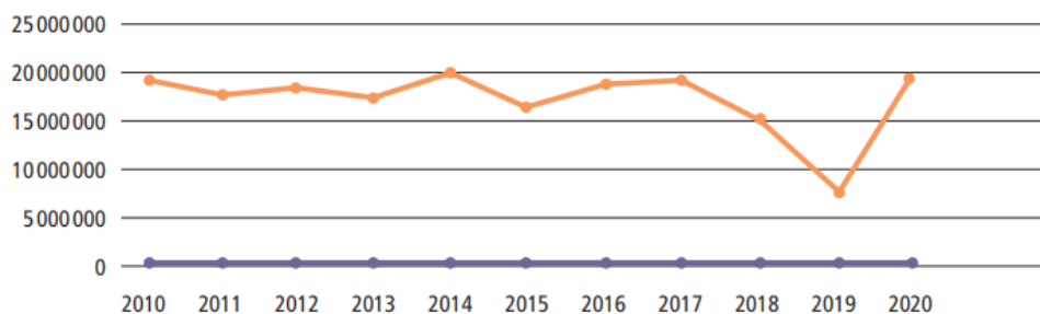
Energieproduktion – Wasserkraft + PV AEM – Meiringen in kWh
